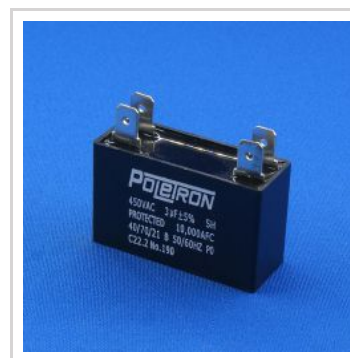
Пусковой конденсатор 3 мкф 450 V CBB61
